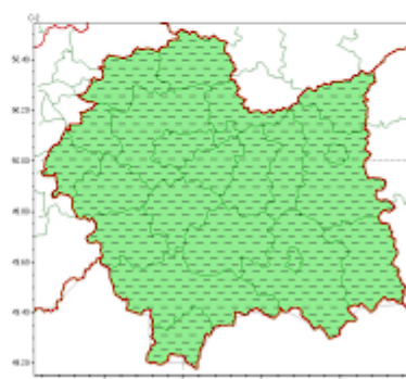
Silny wiatr 2024-09-14 13:01
